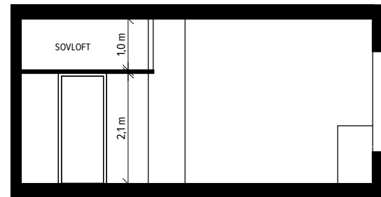
SEKTION A-A
