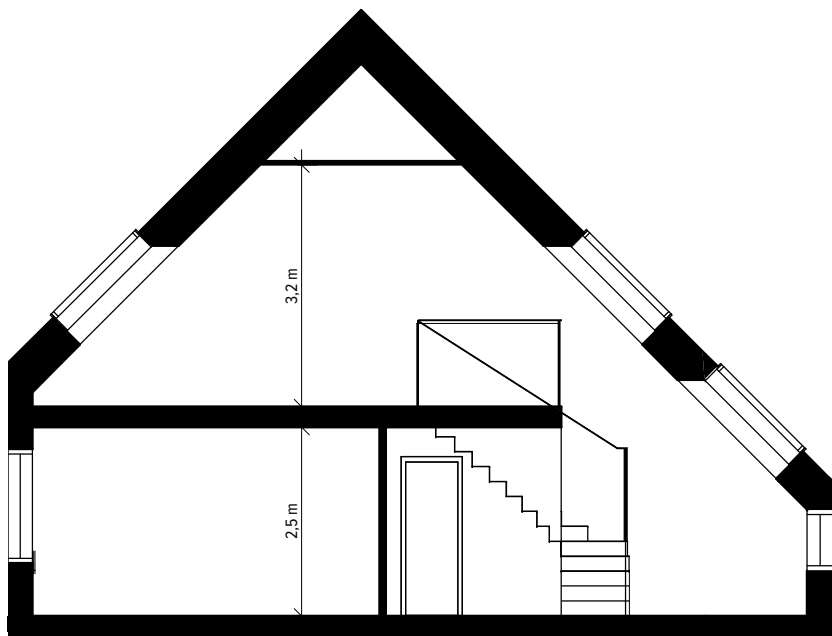
SEKTION A-A
