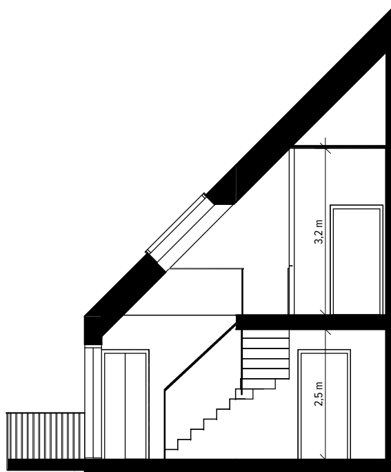
SEKTION A-A
