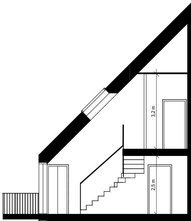
SEKTION A-A
